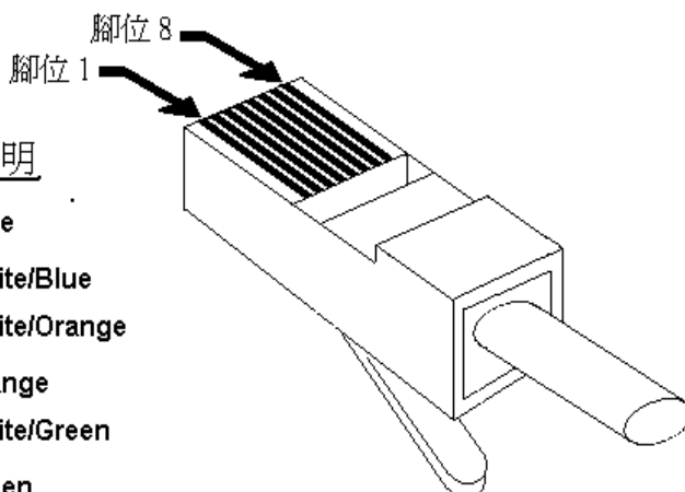
RJ-45 腳位識別圖
